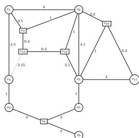
Fig. 8: G
