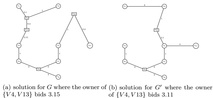
Fig. 9: RZ: solutions
